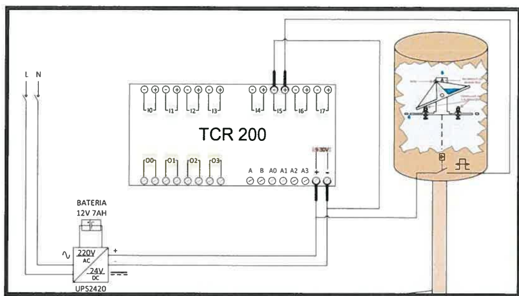
Ejemplo de conexión pluviómetro a equipo de telemetría
